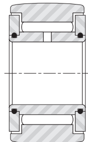
FG/FGL
