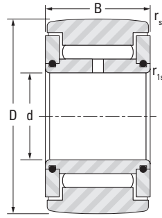
FG, FGL
